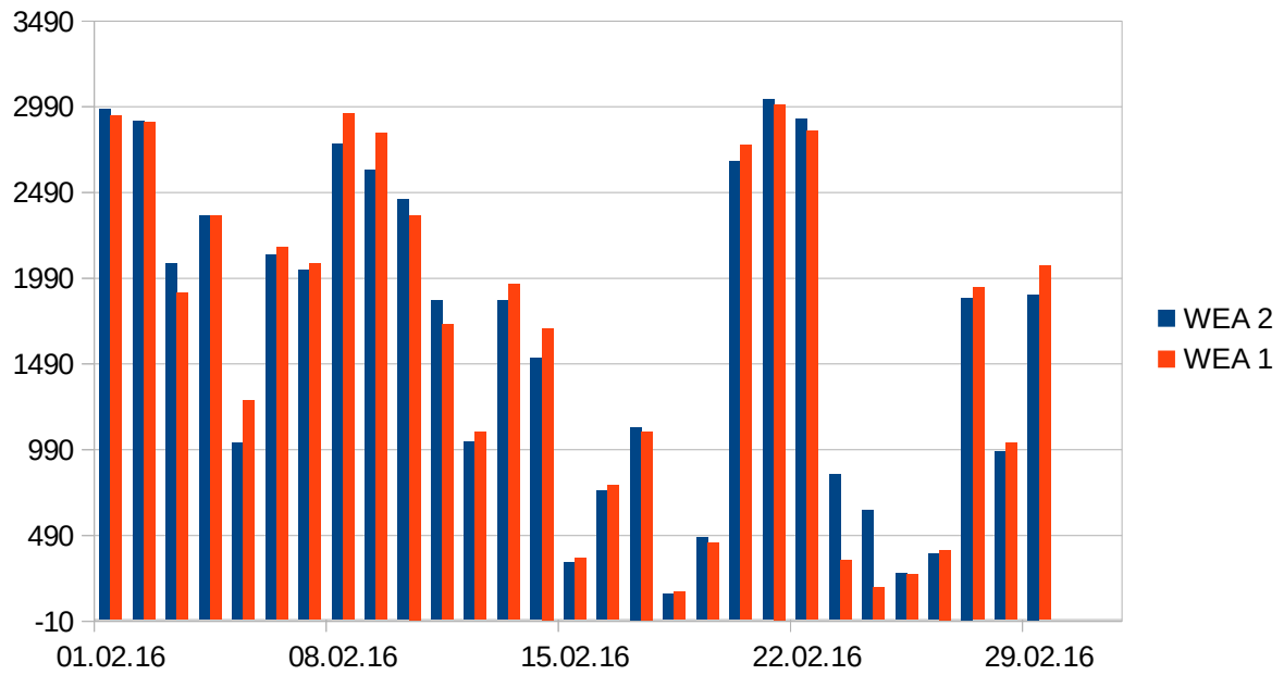
Energieertrag Jahresverlauf
