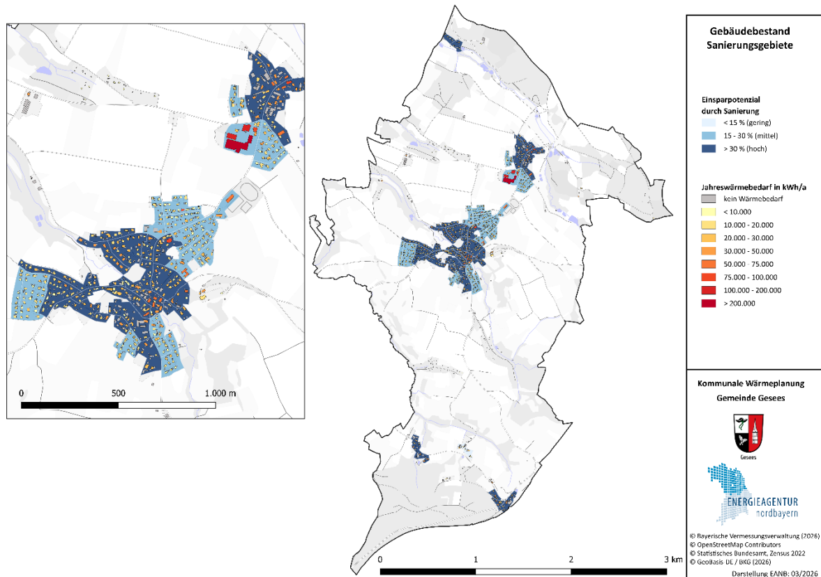
Abbildung 44: Karte Sanierungsgebiete Zielszenario 2045
