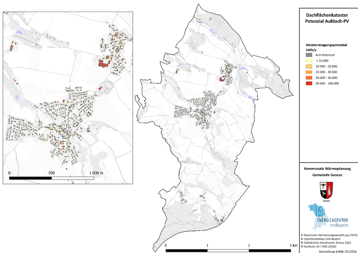
Abbildung 46: Karte Potenzial Aufdach-PV / Dachflächenkataster
