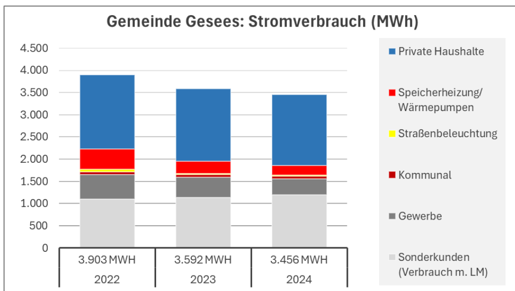
Abbildung 12: Stromverbrauch 2022-2024
