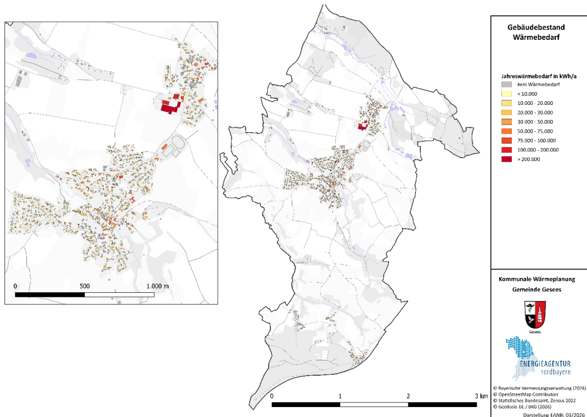
Abbildung 32: Karte Wärmekataster – Jahreswärmebedarf je Gebäude
