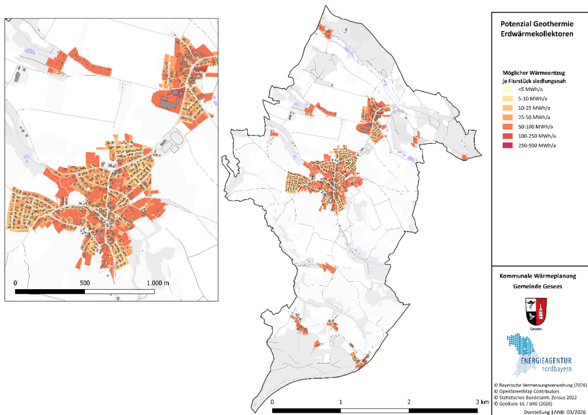
Abbildung 49: Karte Wärmeentzugsenergie Erdkollektoren je Flurstück
